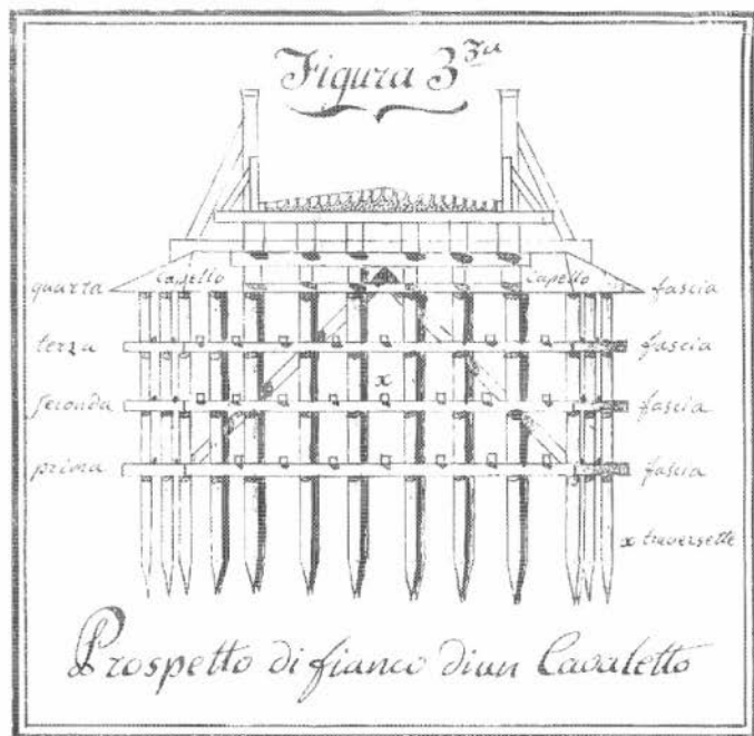
Fig. 2 - "Piano di costruzione del Ponte a bosco progettato sopra la strada di Pinerolo alla Torre varcante il torrente Angrogna all'entrata del capoluogo..."; disegno a china acquerellato, firmato dall'architetto Filippo Ghigliani; 12 novembre 1814 (ASTP 982/1); particolare: "Prospetto di piano di un Cavalletto".
